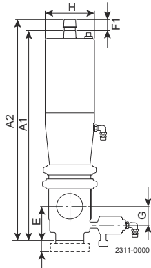
Abbildung 1. a. Absperrventil
